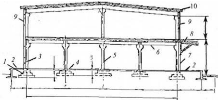
Рис. 2. Конструктивні елементи двоповерхової будівлі складу: 1 — фундамент; 2 — рампа; 3 — стіна; 4 — підлога; 5 — колона; 6 — міжповерхове перекриття; 7 — двері; 8 — піддашшя; 9 — вікно; 10 — верхнє покриття
