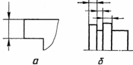
Розміщення стрілок зовні виносних ліній: а — для одного розміру; б — для декількох розмірів.
