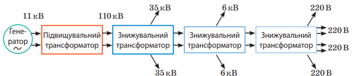
Схема передачі та розподілу енергії в електричній мережі
