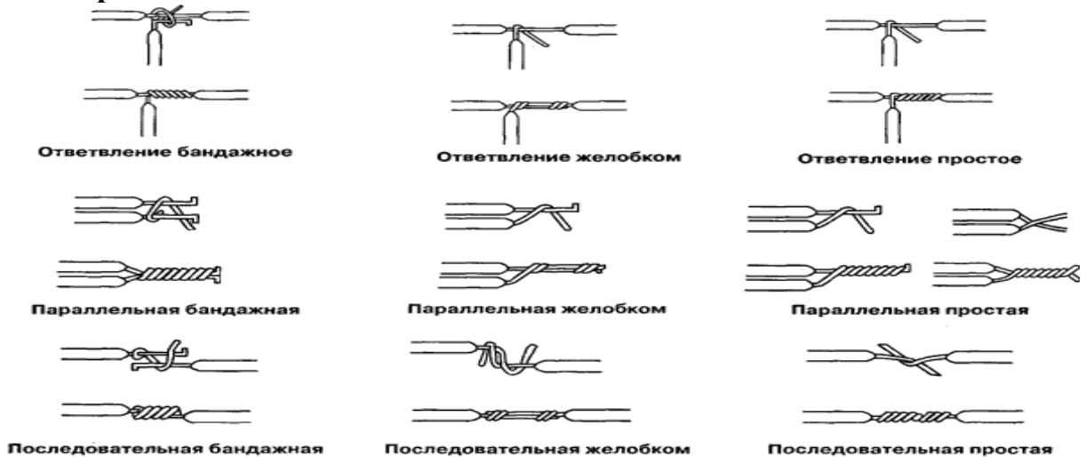
Соединение проводов скруткой
