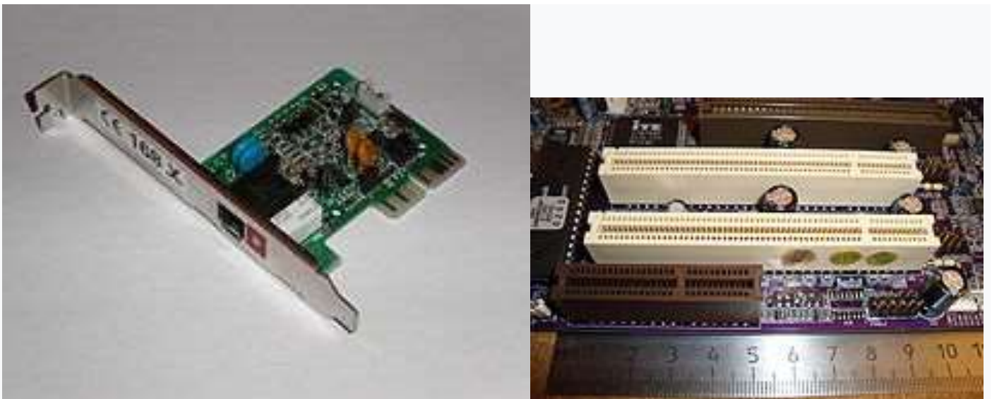
Плата AMR-модема
